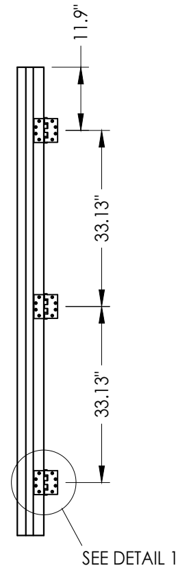
HINGE JAMB
